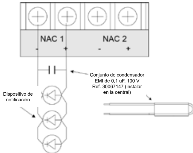
Figure 6. Diagrama de conexión del conjunto del condensador NAC EMI
