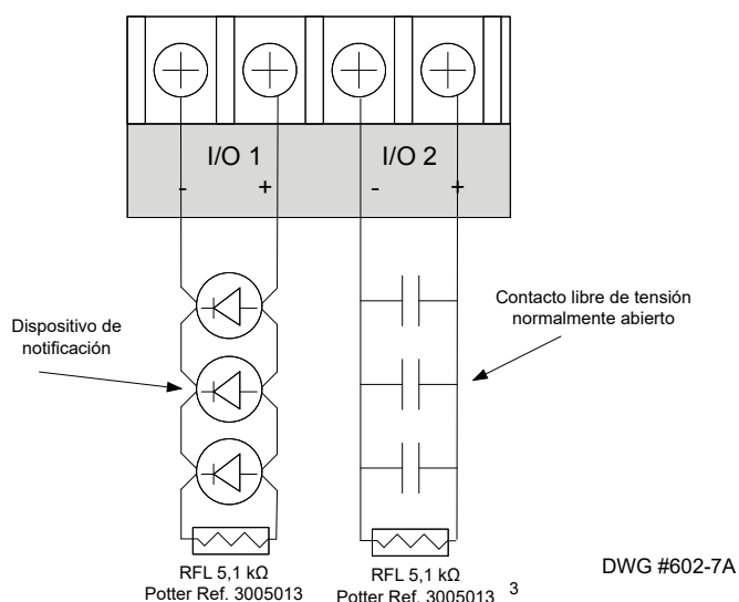
Figure 7. Circuitos de E/S mostrados como NAC Clase B/entrada con contactos libres de tensión
