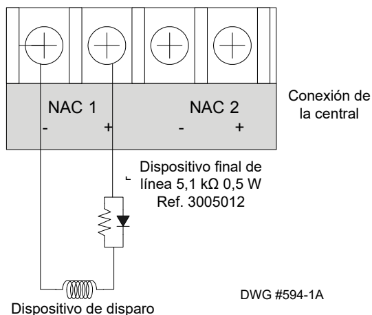
Figure 16. Conexión del circuito de disparo de NAC con conjunto EOLD
