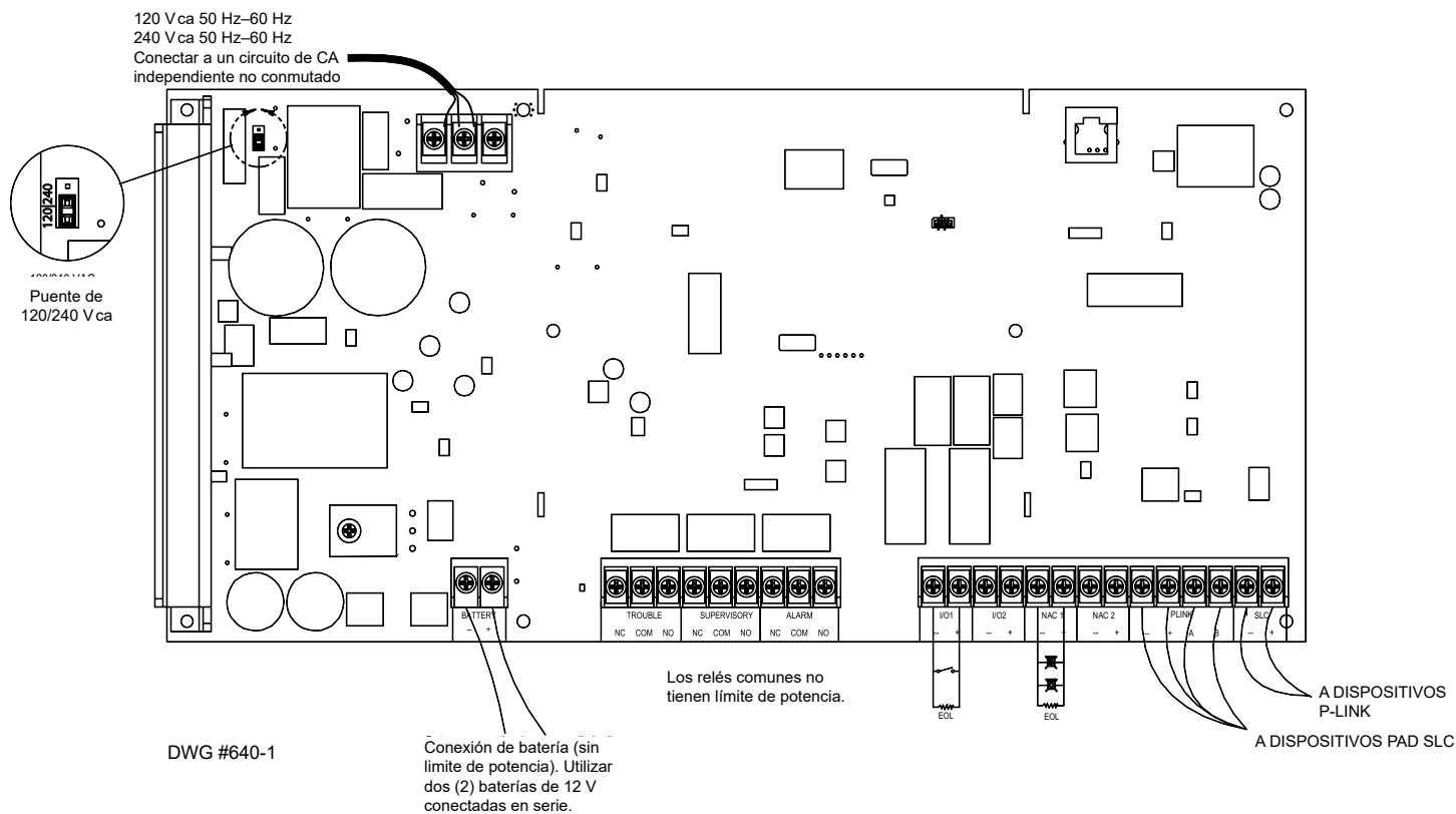
Figure 1. Esquema eléctrico de la central de incendios direccionable IPA-100
