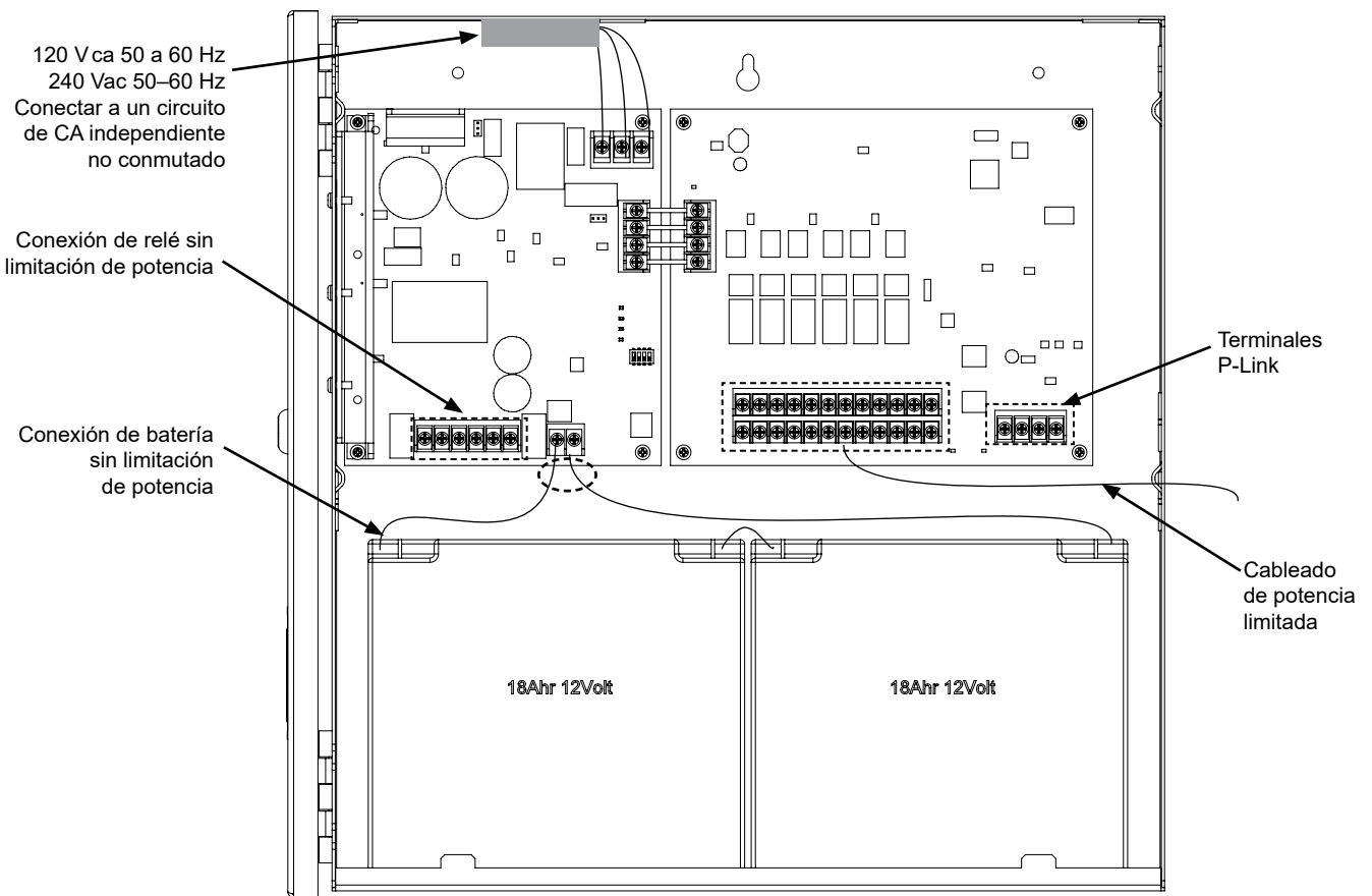
Figure 21. Ejemplo de cableado PSN-1000
