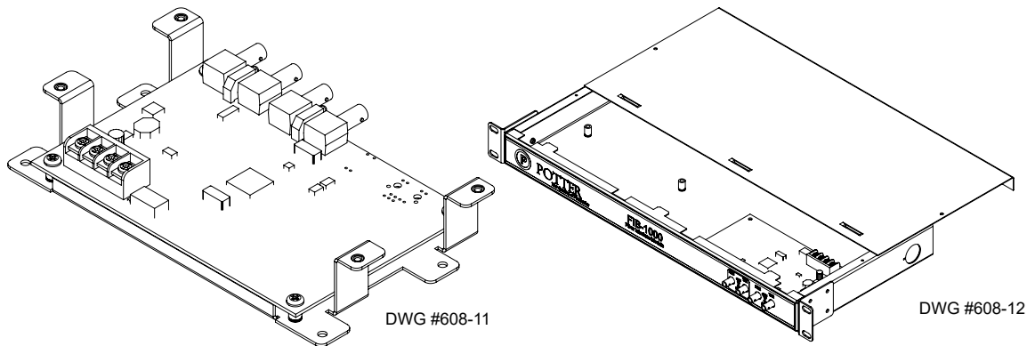
Figure 32. Puente FIB-1000 y FIB-1000RM que muestran el montaje en rack
