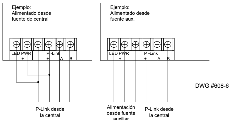
Figure 28. Ejemplos de conexión del DRV-50 desde la central de control o la fuente de alimentación auxiliar
