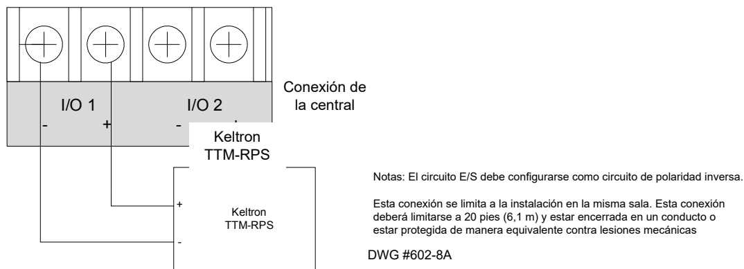
Figure 18. Ejemplo de cableado de circuito de E/S de polaridad inversa
