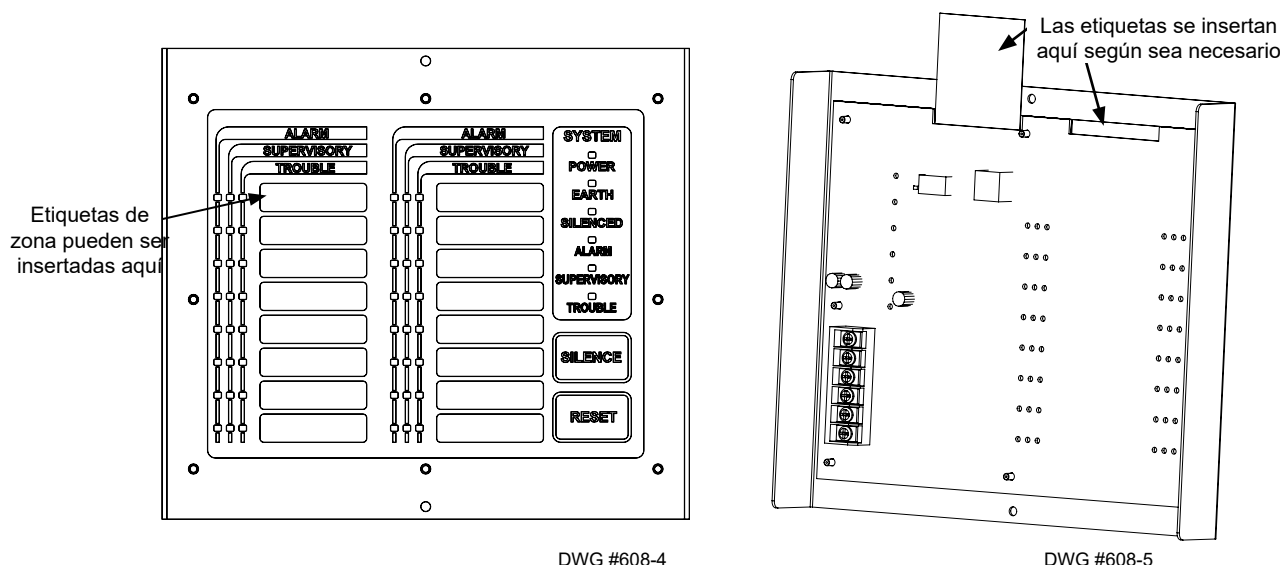
Figure 23. Módulo y placa LED-16/LED-16(F)
