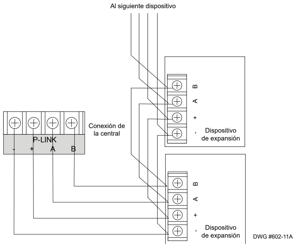
Figure 14. Ejemplo de cableado P-Link Clase B
