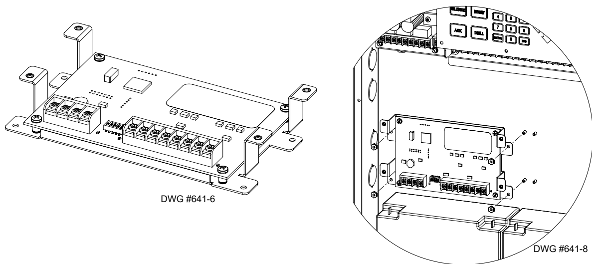
Figure 34. Se muestran la placa MC-1000 Multi-Connect y el MC-1000 instalados en el armario IPA-4000
