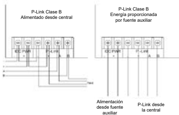
Figure 37. Conexión IDC-6 Clase B
