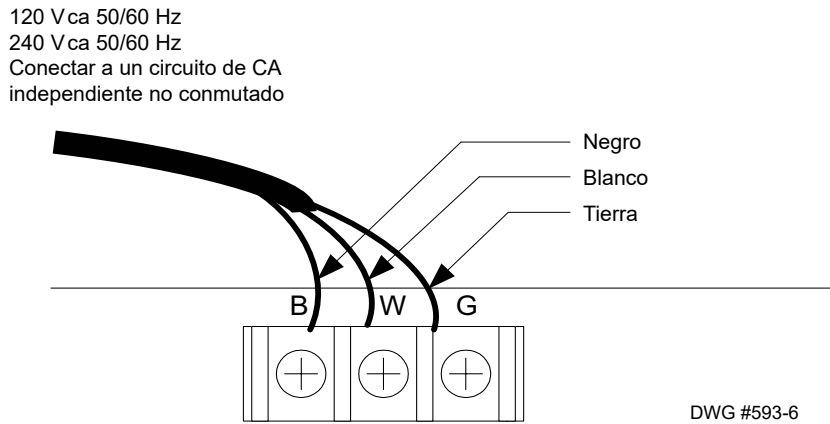
Figure 2. Circuito de alimentación principal
