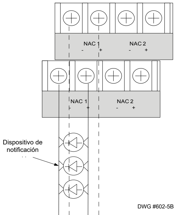
Figure 4. Conexión NAC Clase B
