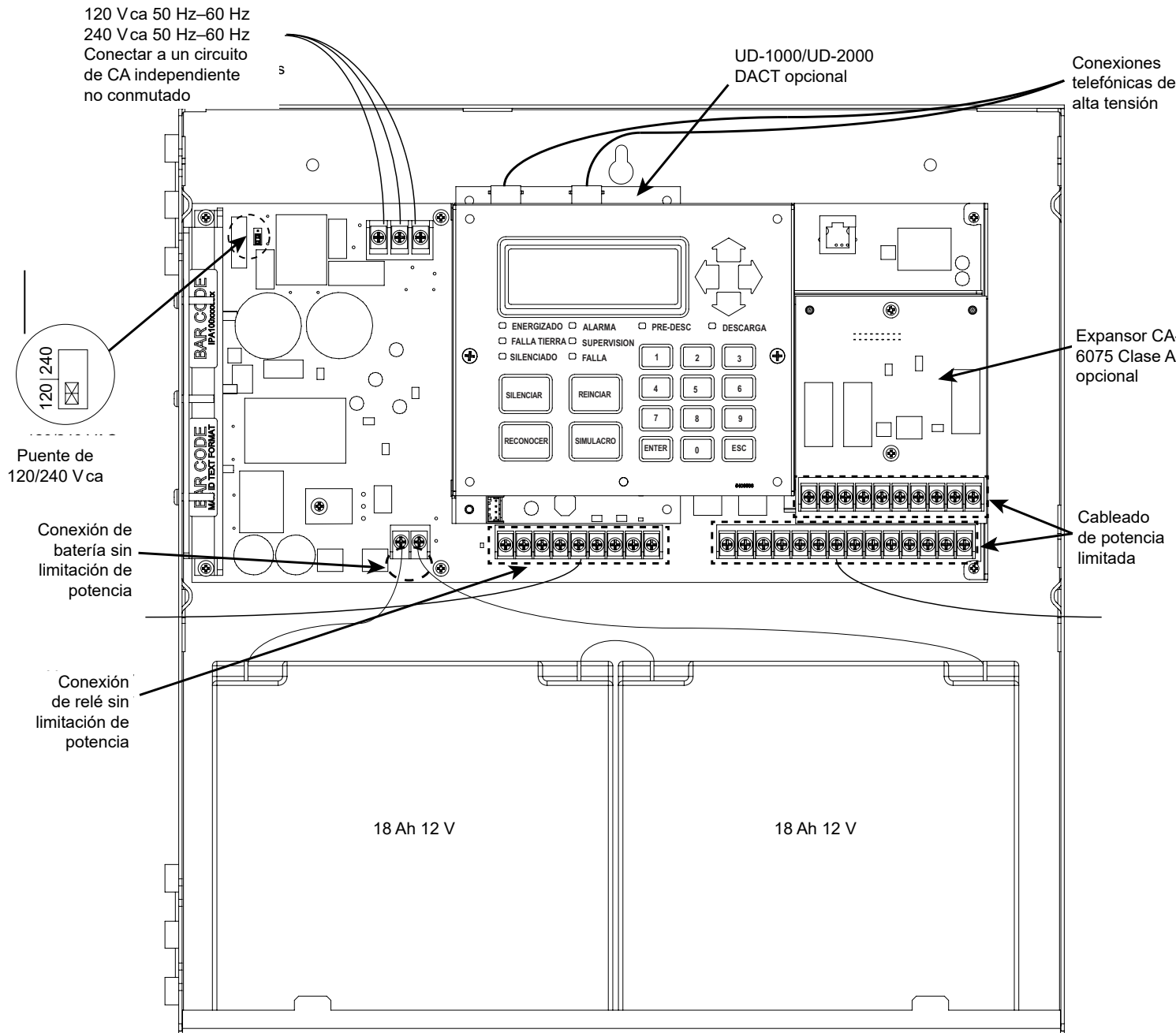
Figure 20. Ejemplo de ruta de cables de la central
