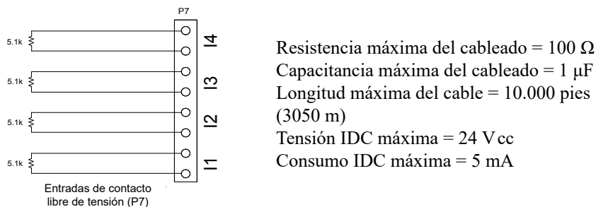
Figure 27. Conector "P7" de entrada con contactos libres de tensión DRV-50
