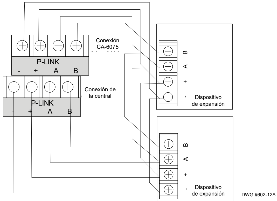
Figure 15. Ejemplo de cableado P-Link Clase A que requiere un CA-6075
