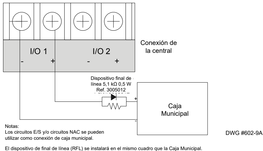
Figure 17. Ejemplo de cableado de caja municipal
