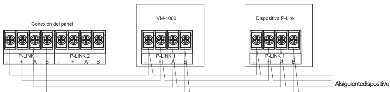
Figura 42. Ejemplo de cableado VM-1000 P-Link Clase B
