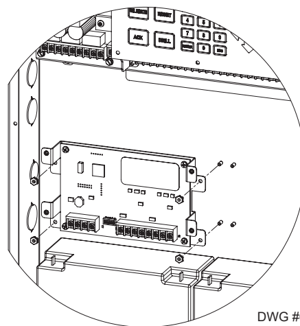
Figura 34. Se muestran la placa MC-1000 Multi-Connect y el MC-1000 instalados en el armario IPA-4000
