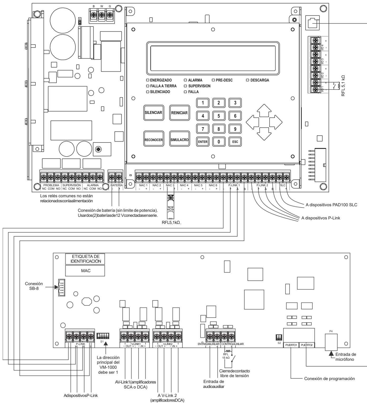
Figura 40. Esquema de conexión de la central de incendios direccionable IPA-4000 con voz inteligente
