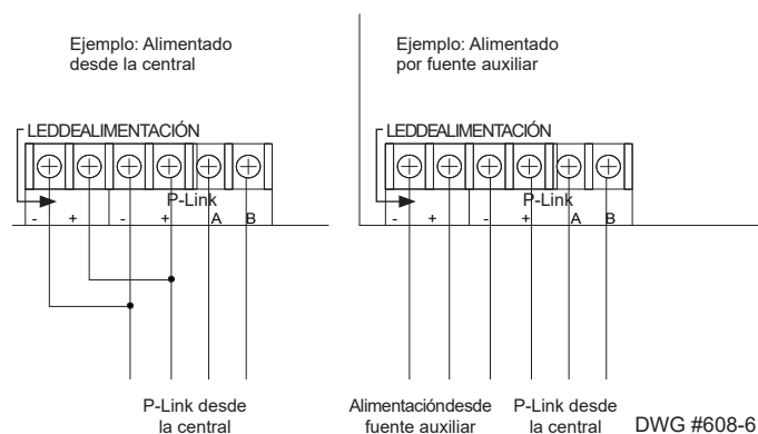
Figura 24. Ejemplos de cableado de un módulo LED-16/LED-16(F) a la central de incendios o fuente de alimentación auxiliar
