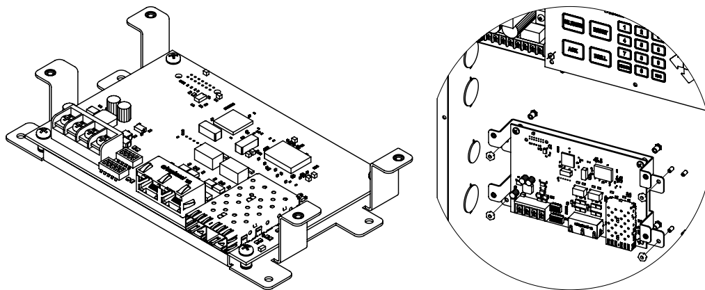
Figura 39. Fibra de tarjeta de red NCF-1000
