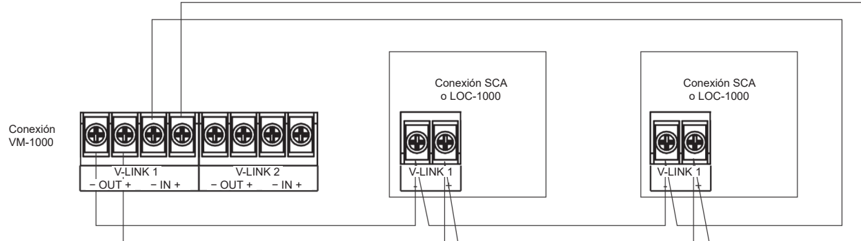
Figura 45. Ejemplo de cableado VM-1000 V-Link Clase A
