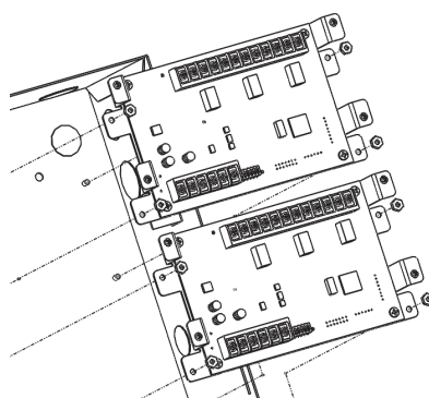
Figura 35. Expansor de circuito del dispositivo iniciador IDC-6 e instalación del IDC-6
