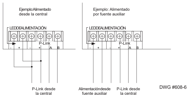
Figura 28. Ejemplos de cableado del DRV-50 desde la central de incendios o la fuente de alimentación auxiliar
