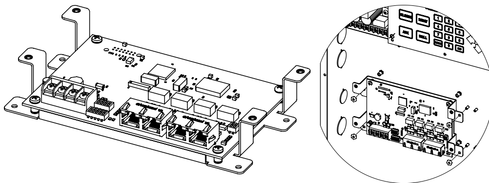
Figura 38. Tarjeta de red NCE-1000
