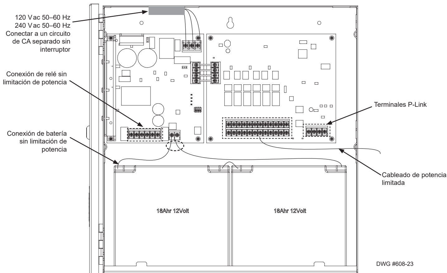
Figura 21. Ejemplo de cableado PSN-1000
