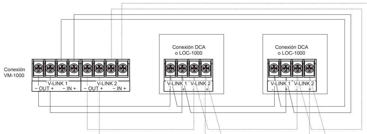
Figura 47. Ejemplo de cableado VM-1000 V-Link 1 y 2 Clase A
