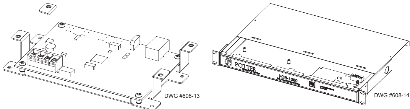
Figura 31. Puente FCB-1000 y FCB-1000RM que muestra el montaje en bastidor
