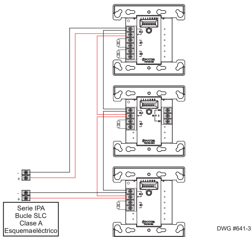
Figura 9. Ejemplo de protocolo PAD de SLC como Clase A
