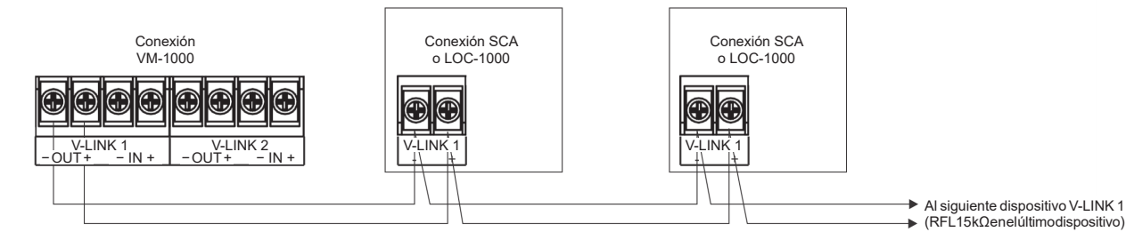
Figura 44. Ejemplo de cableado VM-1000 V-Link Clase B
