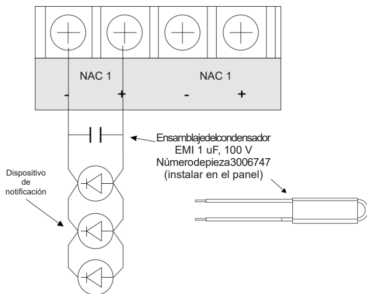
Figura 6. Diagrama de cableado del conjunto del condensador NAC EMI
