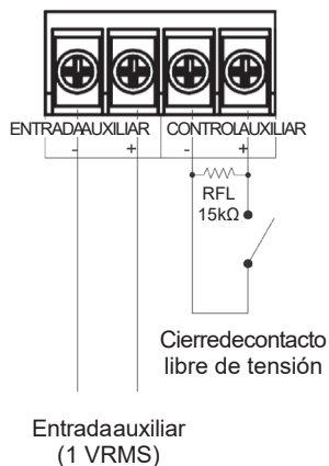
Figura 48. Entrada auxiliar VM-1000
