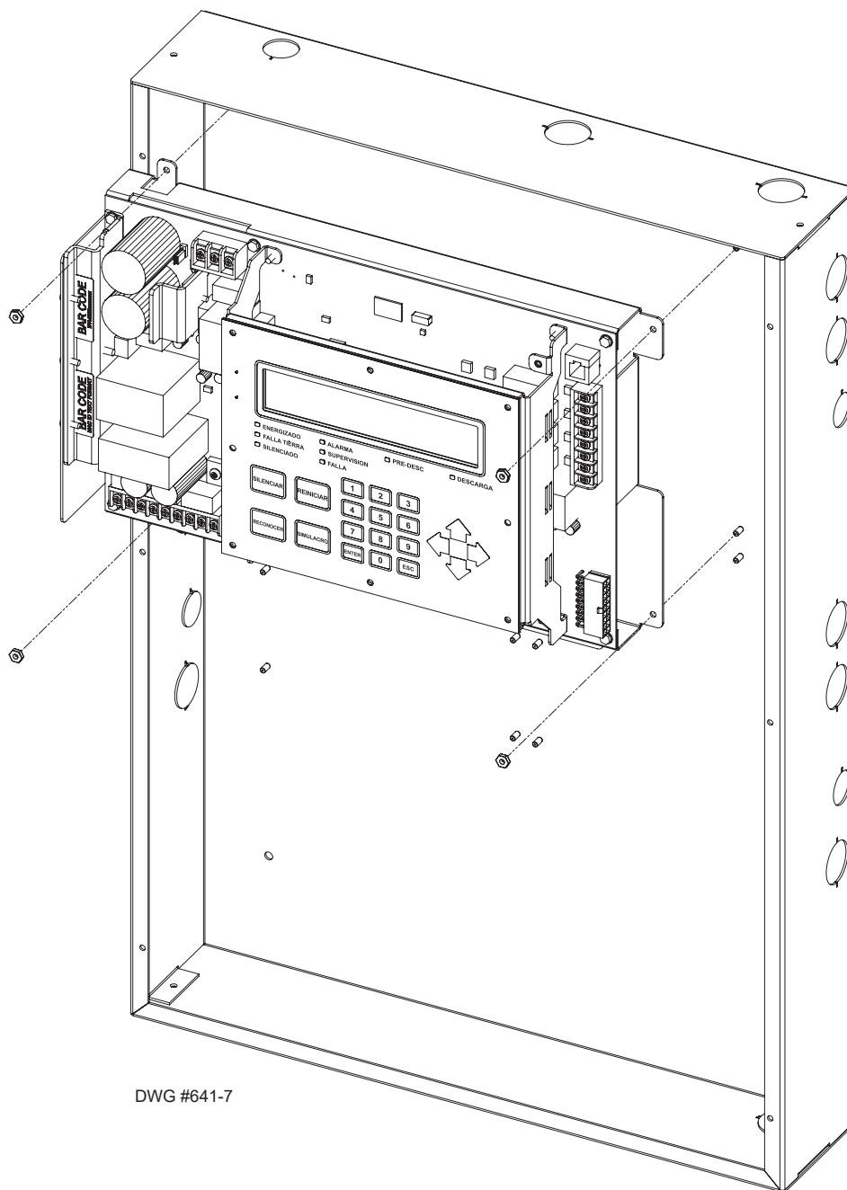
Figura 52. Armario IPA-4000 que muestra el ensamblaje de la placa de circuito
