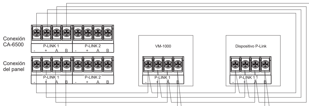
Figura 43. Ejemplo de cableado VM-1000 P-Link Clase A
