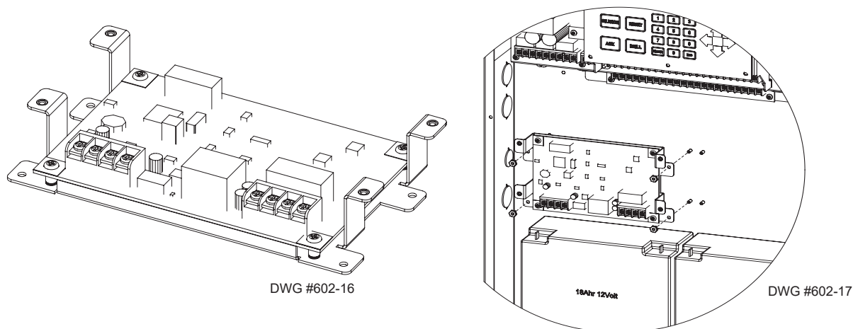
Figura 22. Placa PAD100-SLCE/Protocolo Nohmi SLCE-127 y se muestra instalada en el armario IPA-4000
