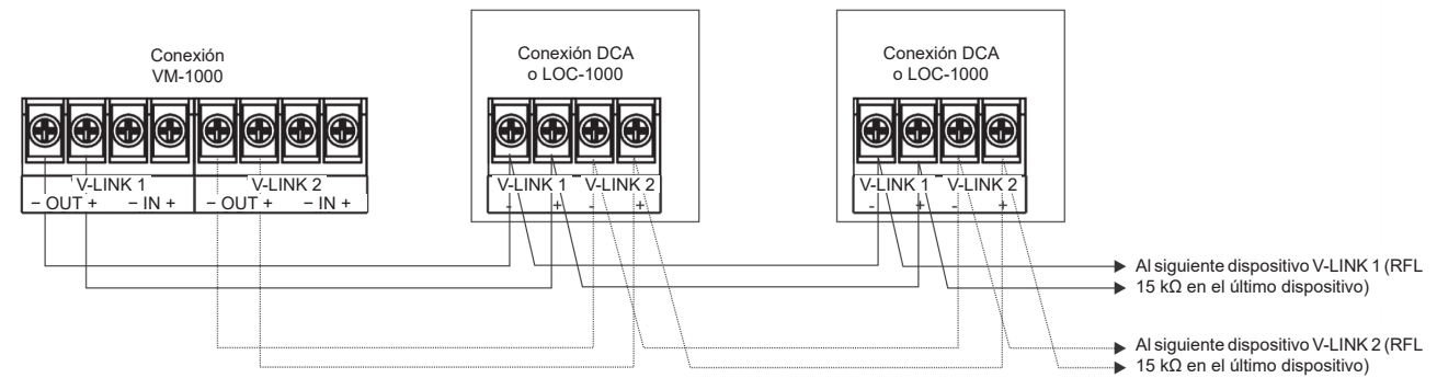
Figura 46. Ejemplo de cableado VM-1000 V-Link 1 y 2 Clase B
