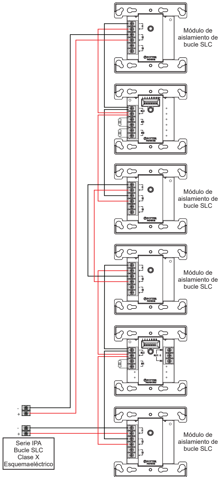
Figura 8. Protocolo PAD Clase X que muestra los PAD100-IM instalados
