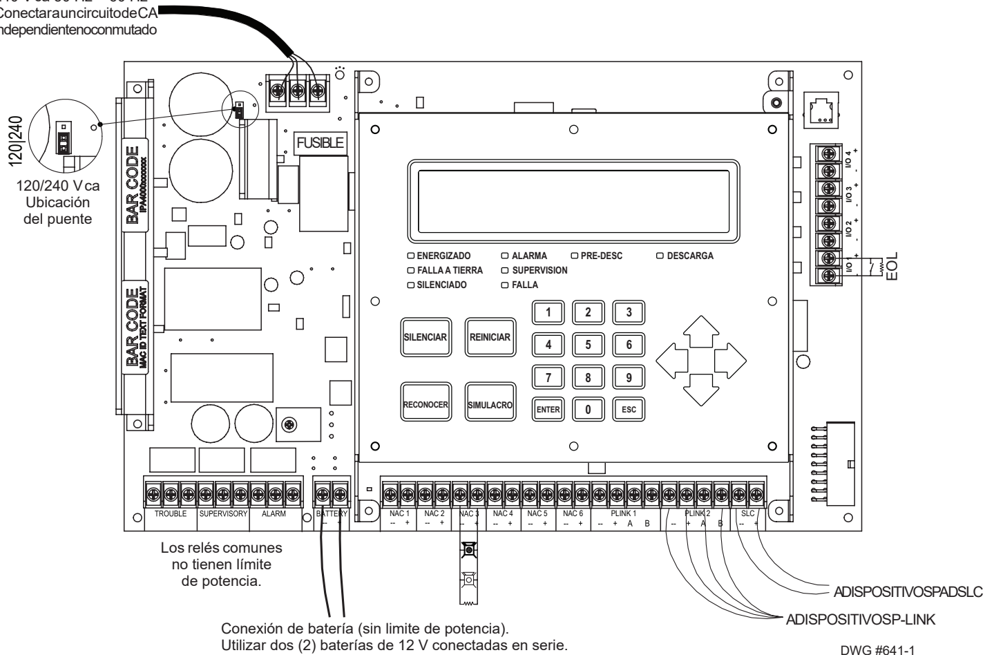
Figura 1. Esquema de conexión de la central de incendios direccionable IPA-4000 con voz inteligente
