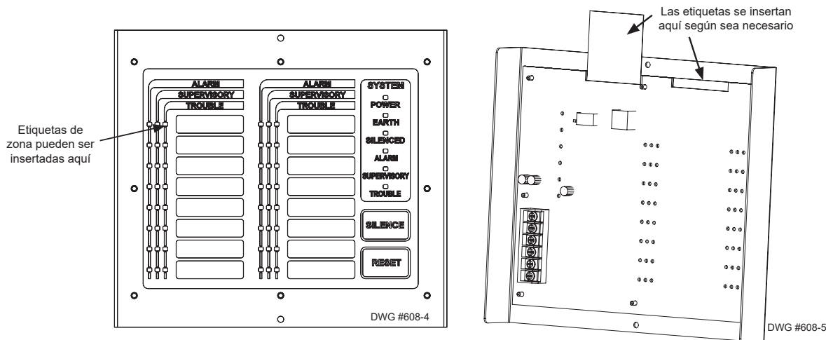
Figura 23. Módulo y placa LED-16/LED-16(F)
